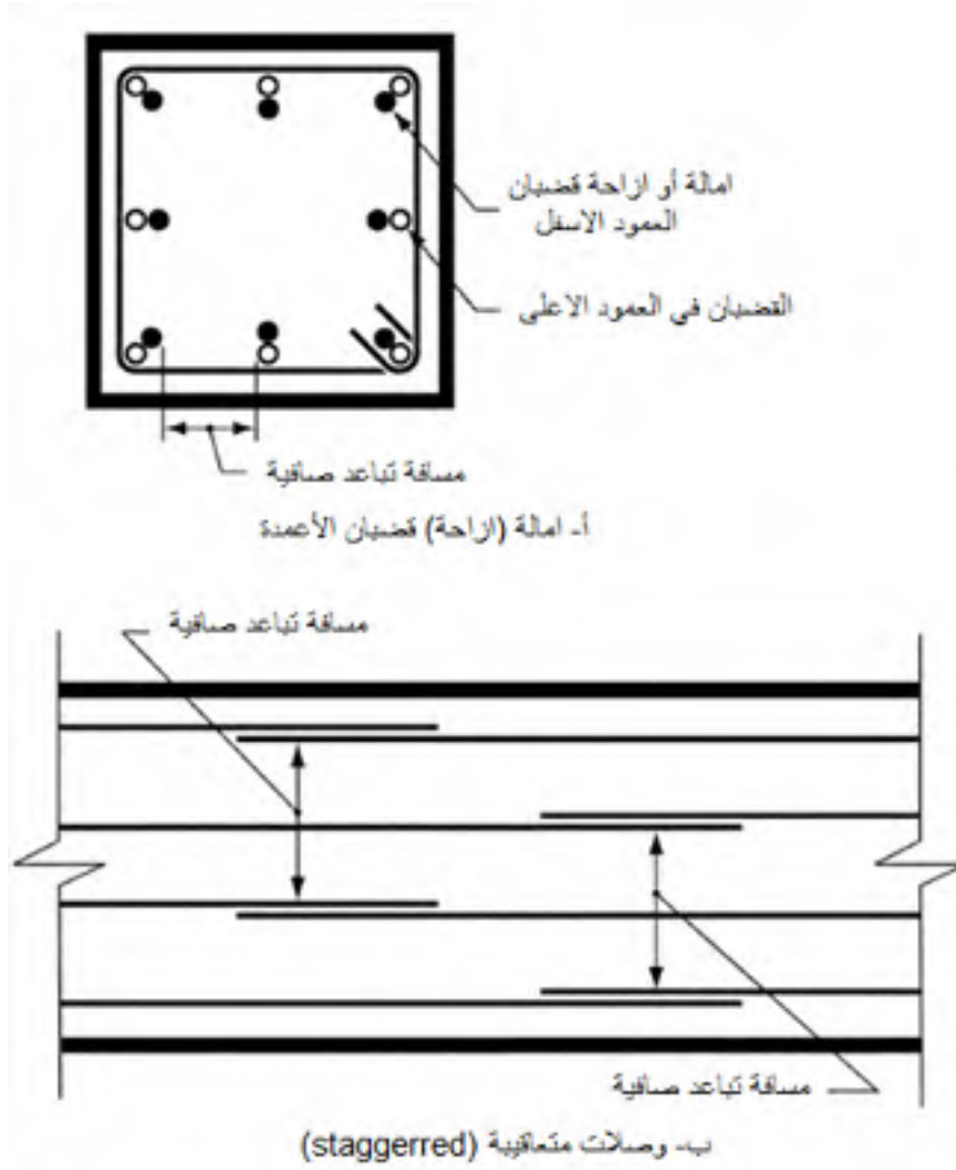
شكل (9-12) المسافة الصاقية بين القضبان الموصولة
