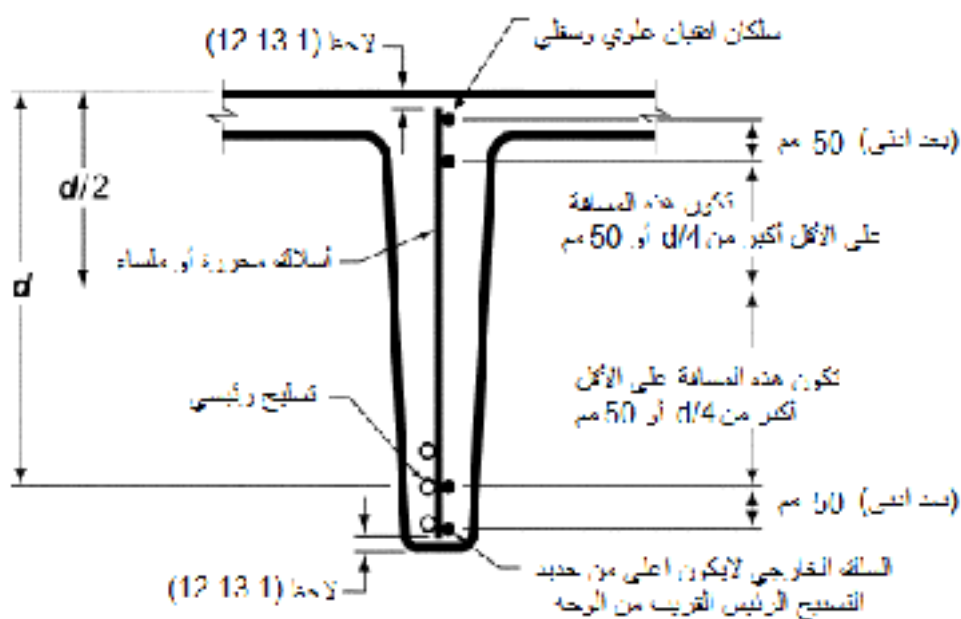
شكل (9-11) تثبيت تسليح القص على شكل ساق مفردة مصنعة من شبكات الأسلاك الملحومة
